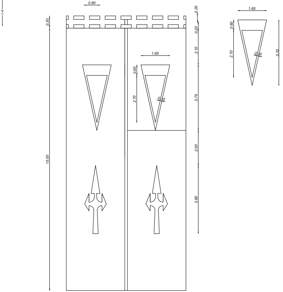
DETALLE DEMARCACIÓN CEDA EL PASO
