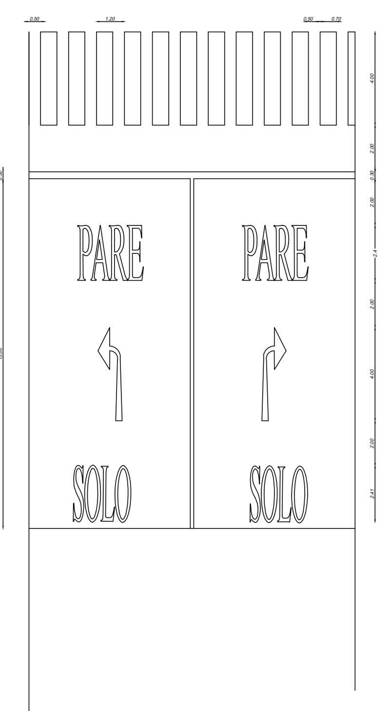
DETALLE DEMARCACIÓN PARE
