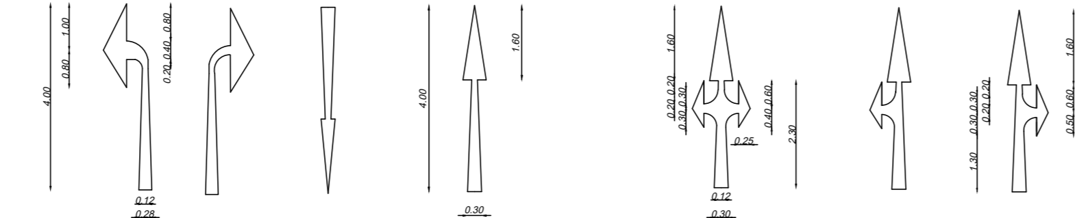
DETALLE DEMARCACIÓN SEÑALES DE DIRECCIÓN
